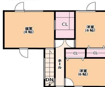
2階平面図
